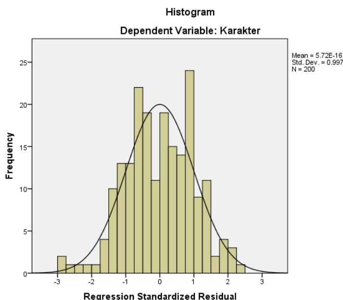
Gambar 1. Grafik histogram uji normalitas antara variabel penerapan nilai-nilai Kristiani (X) terhadap variabel Karakter (Y)
