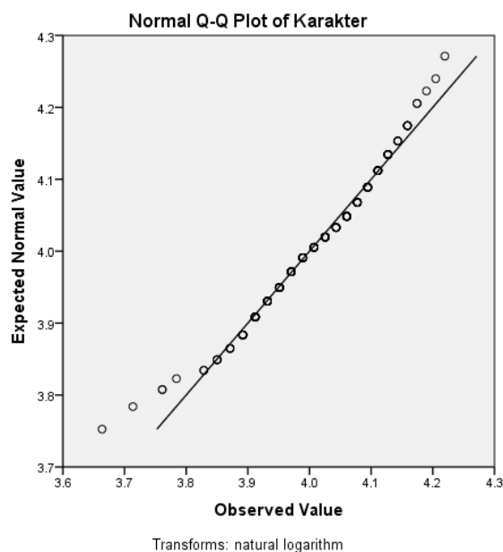
Gambar 2. Grafik Q-Q Plot uji normalitas antara variabel penerapan nilai-nilai Kristiani (X) terhadap variabel Karakter (Y)
